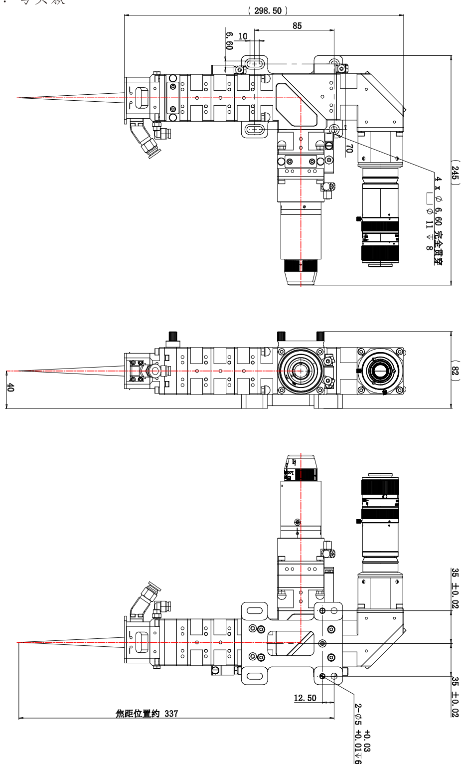
外形尺寸图：弯头款
